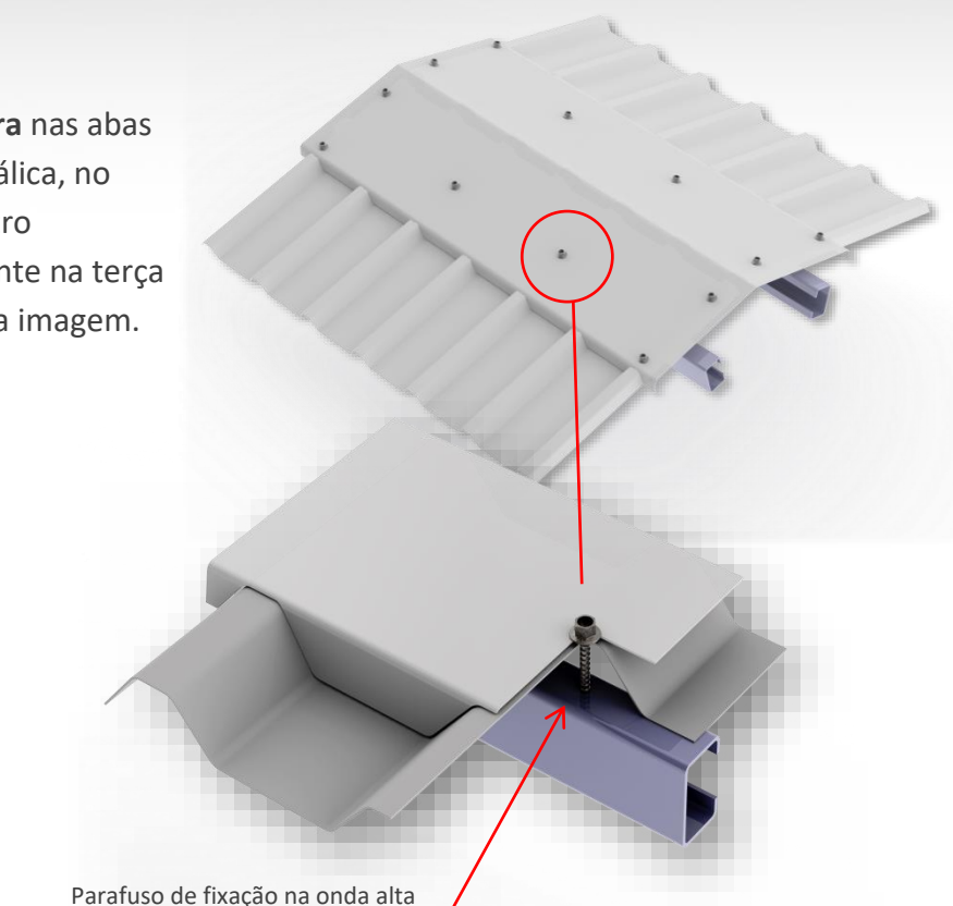
Parafuso de fixação na onda alta
